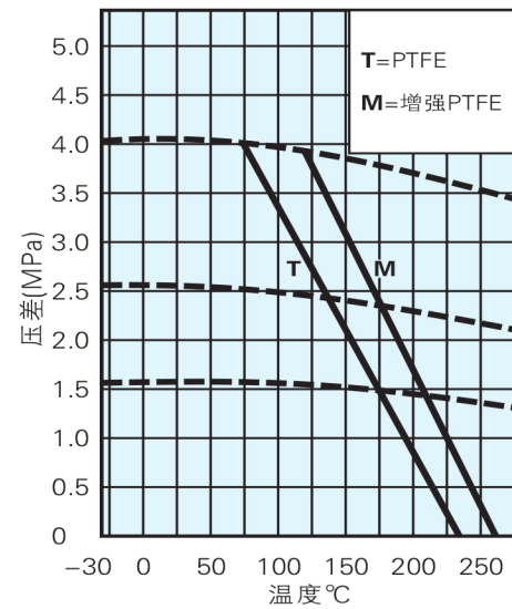
DN150~DN300
