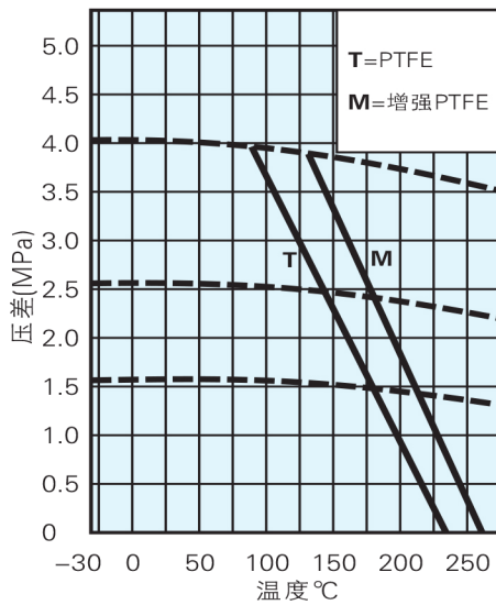
DN80~DN125
