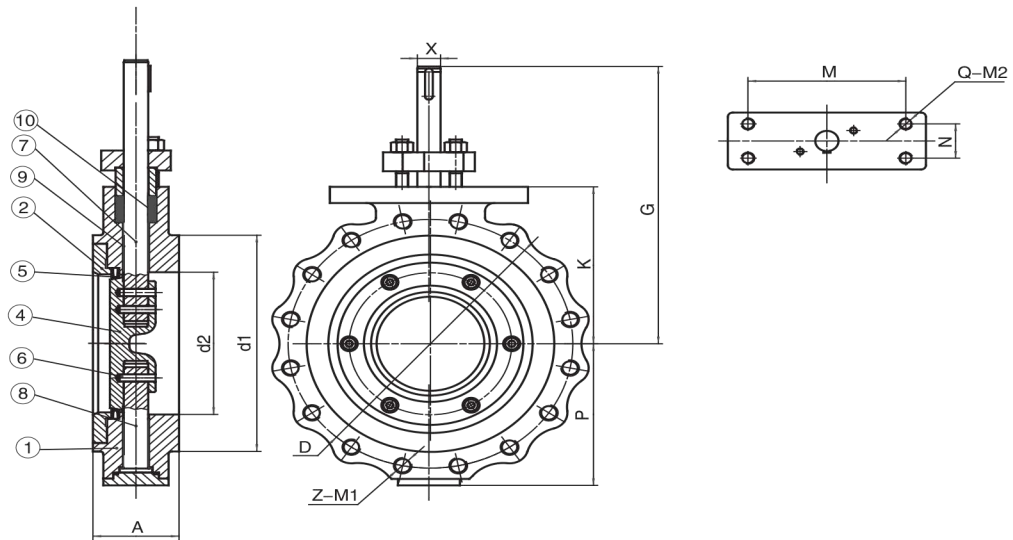
HP8-150L 凸耳式蝶阀尺寸 CLASS 150
