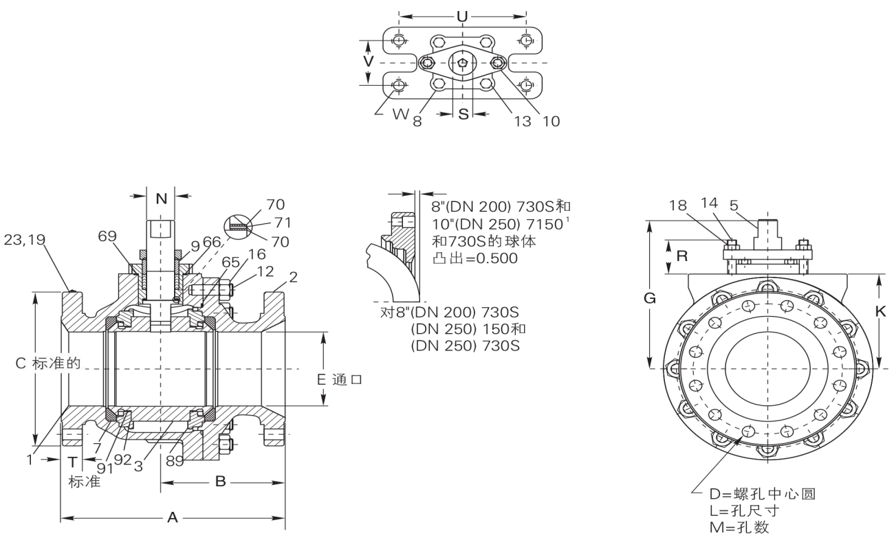
10"(DN 250)7150系列，8"和10"(DN 200和250)7300和730S
