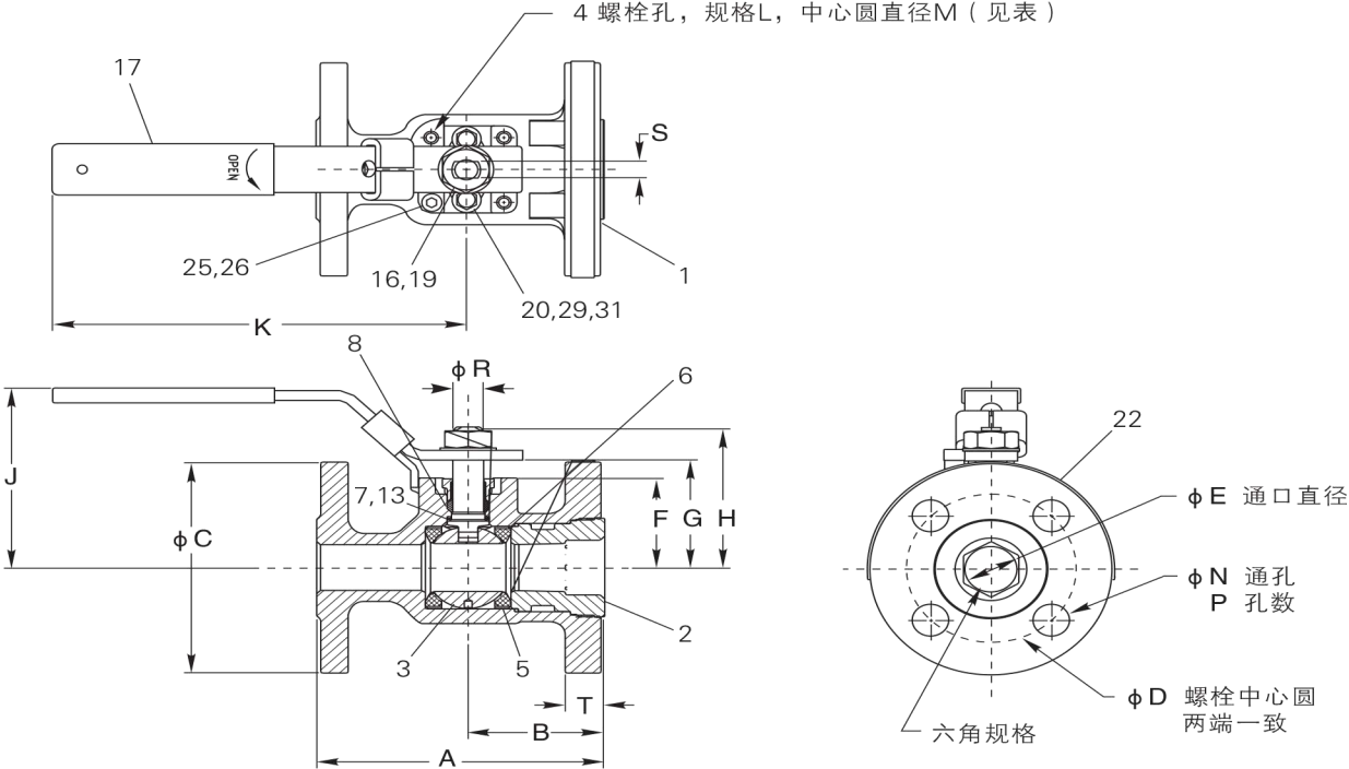
150级7150和300级7300与730S法兰连接球阀
