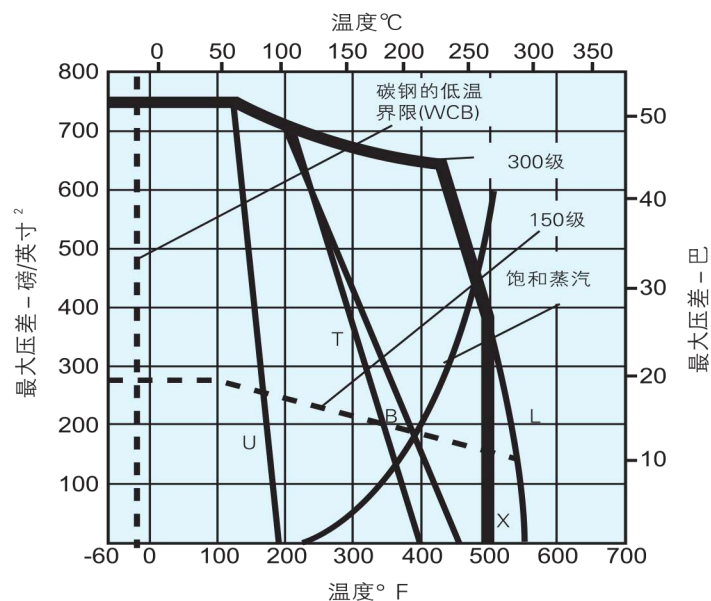
1/2"-2" (DN15-50)缩口
