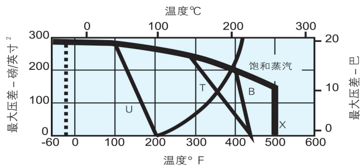
8" (DN200)缩口, 非固定球
