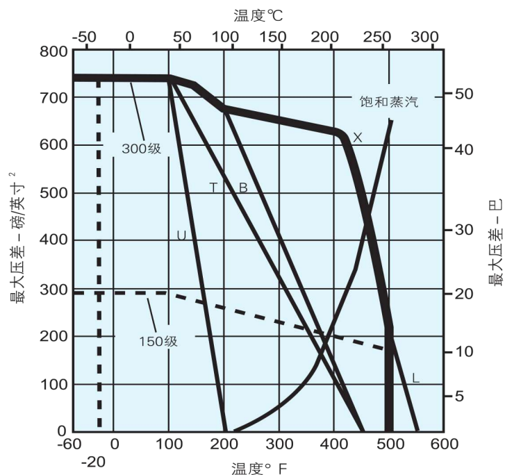
3"-6" (DN80-150)缩口
