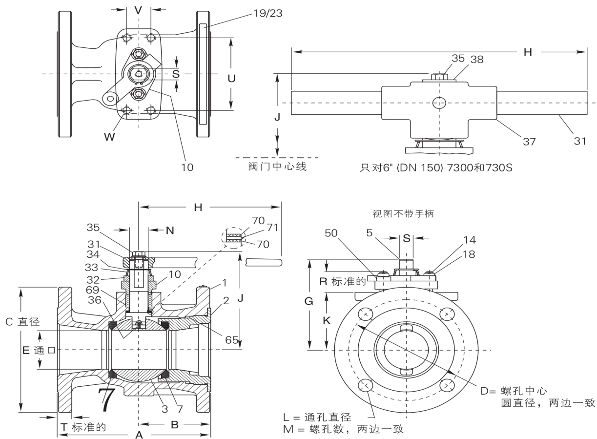
3"---6" (DN80-150)150级7150和300级7300与730S(非固定球)法兰连接阀门
