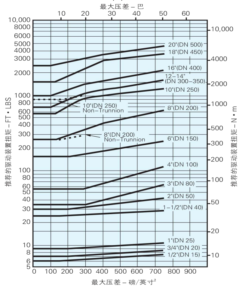
UHMW (U)密封座阀门
