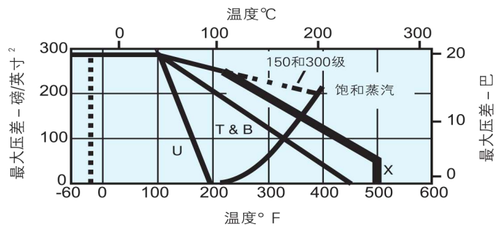
8" (DN200)全口径, 非固定球
