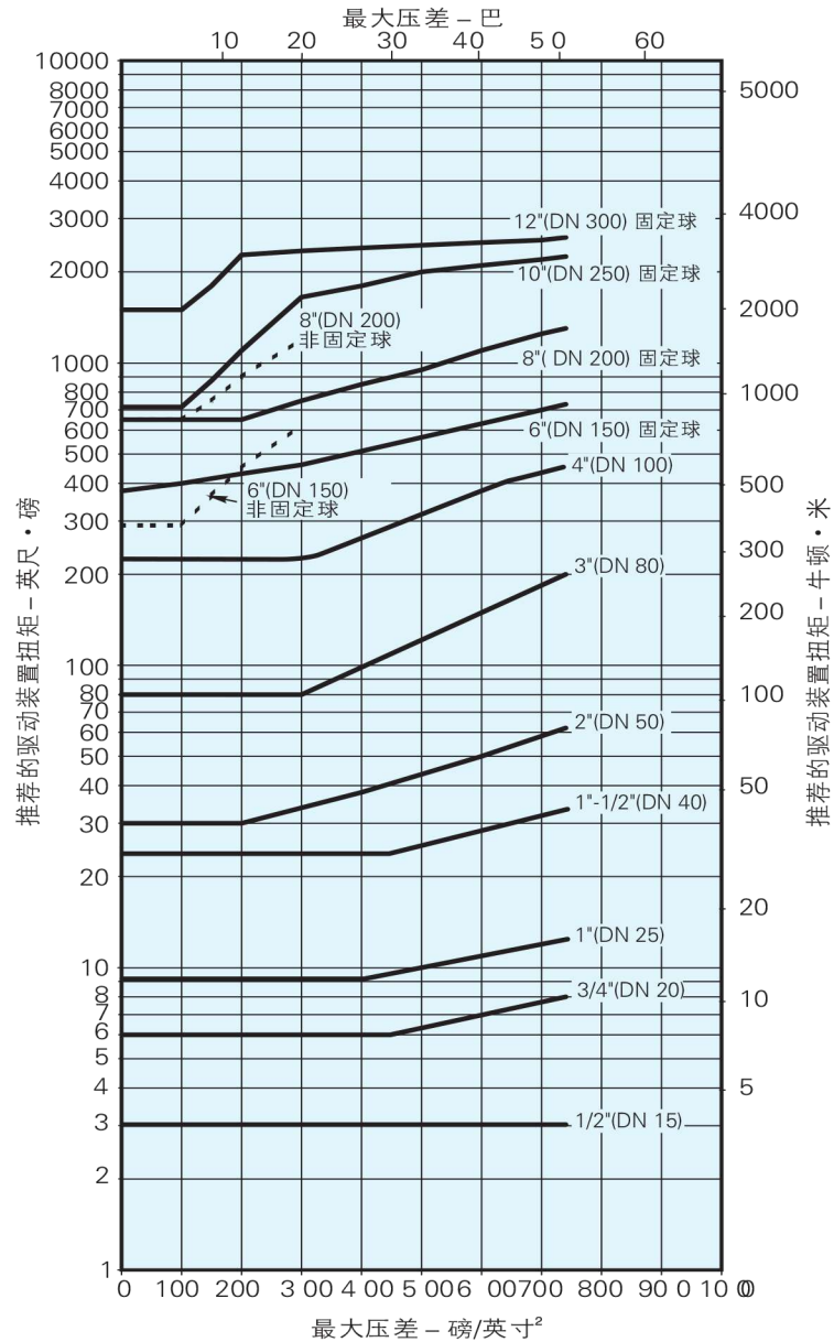
SPTFE (X)密封座阀门, 1/2"-12" (DN15-300)
