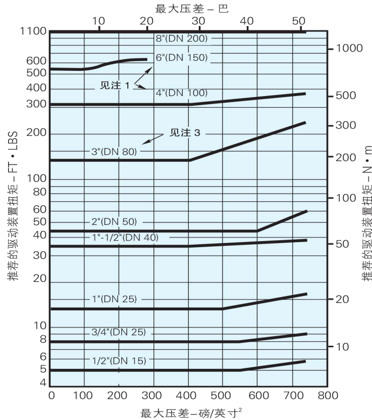
PFA (B)密封座阀门, 1/2"-8" (DN15-200)
