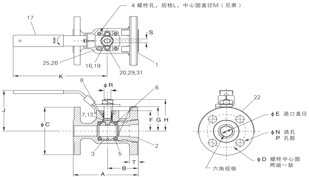
1/2"-1-1/2" (DN15-40)150级9150和300级9300阀门
