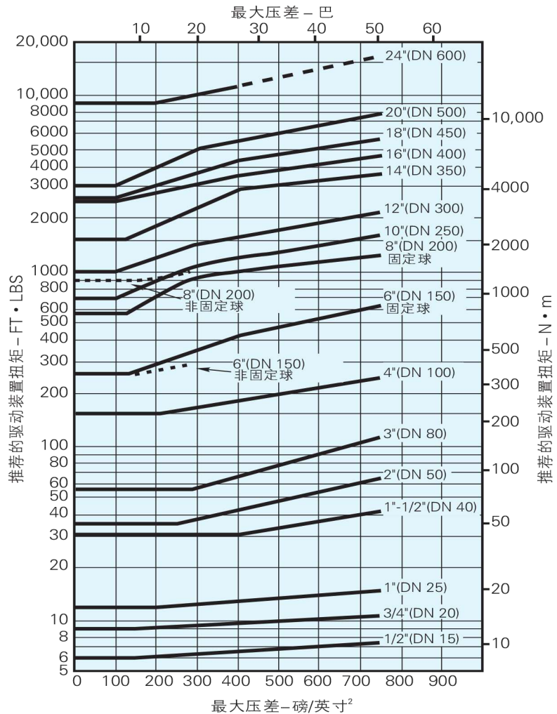
UHMW (U)密封座阀门
