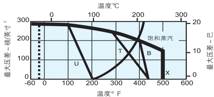
6" (DN150)全口径, 非固定球
