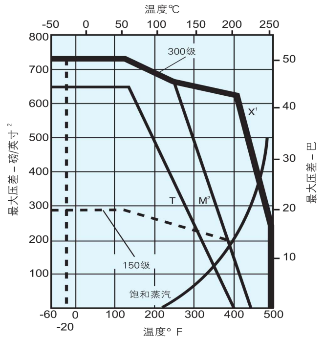
6"-24" (DN150-600)全口径, 固定球
