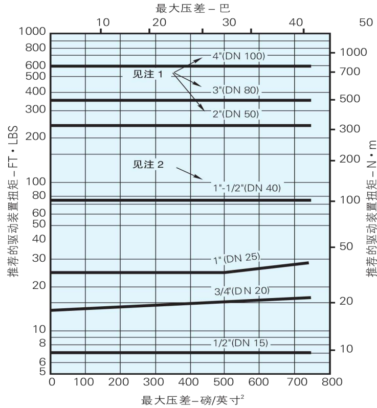
Peek (L)密封座阀门, 1/2"-6" (DN15-150)
